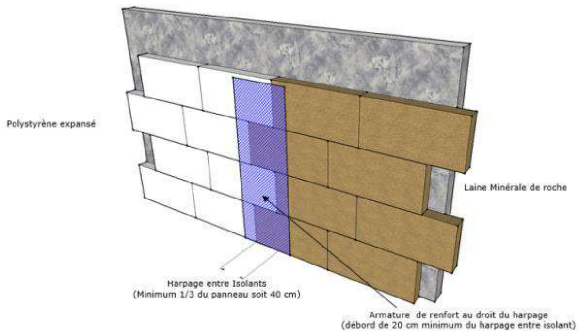
Figure 2a : harpage des isolants
