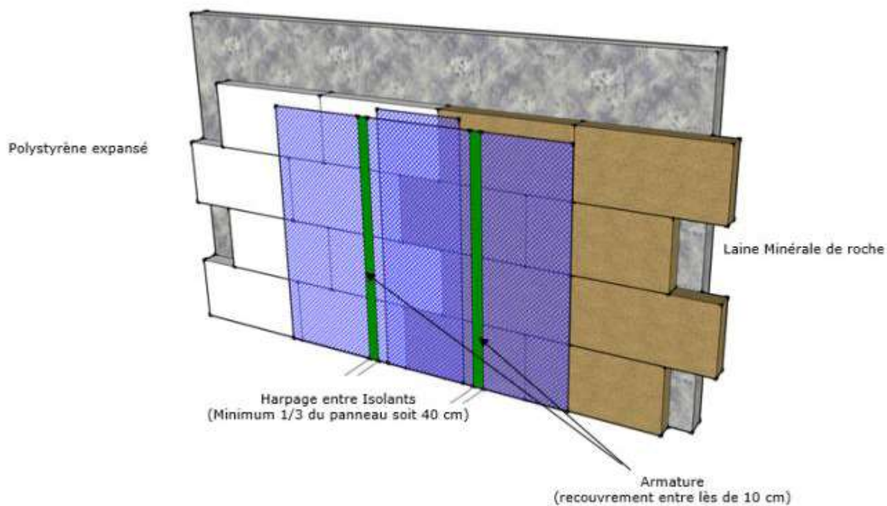
Figure 2c : Mise en place de l'armature en partie courante lors d'une mixité des isolants
