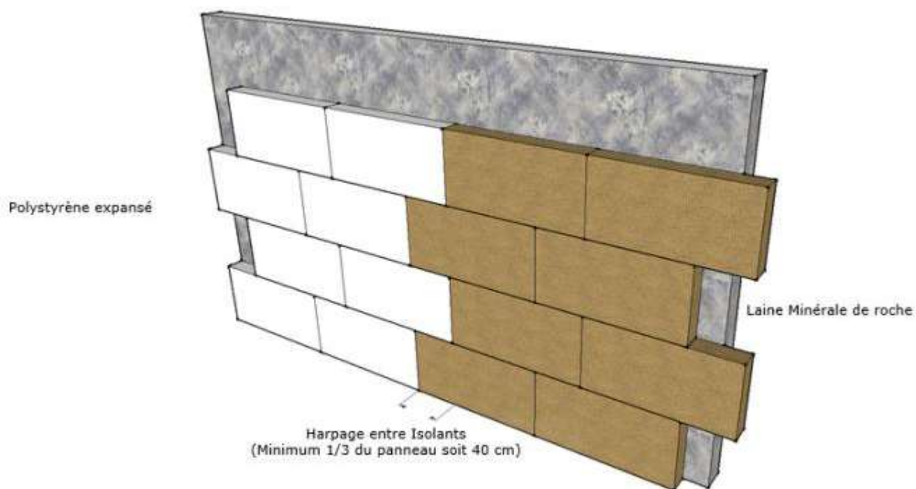
Figure 2a : harpage des isolants
