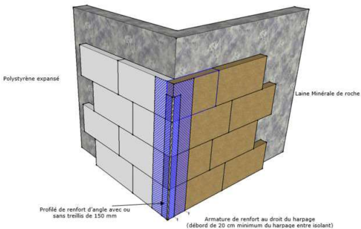
Figure 3 : Mixité des isolants – traitement des angles
