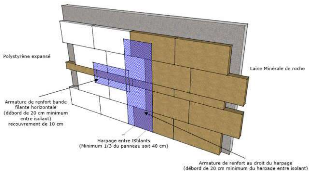
Figure 4 : Mixité des isolants – pose des bandes filantes
