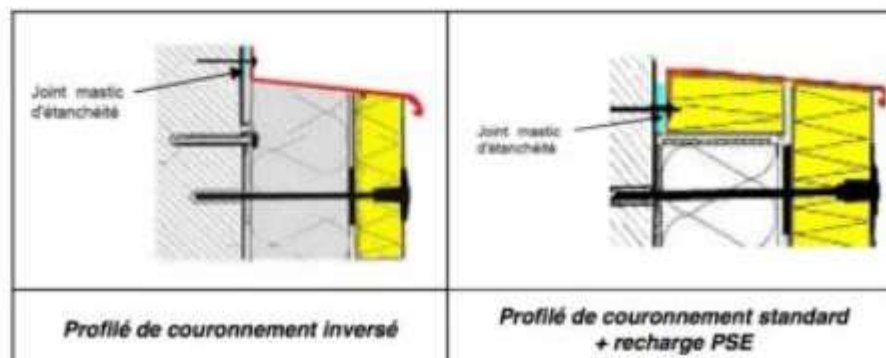
Figure 6 : traitement des points singuliers en surisolation
